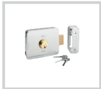
DU.V90 Elettroserratura 12 Vac/dc orizzontale fornita con piastra d'incontro e doppio cilindro. Consente sblocco interno/esterno.
